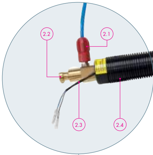
Figure 2 : Connexion du faisceau
